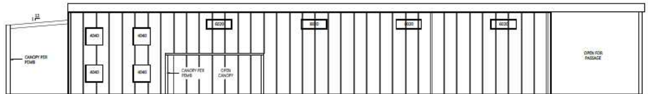
RIGHT ELEVATION
